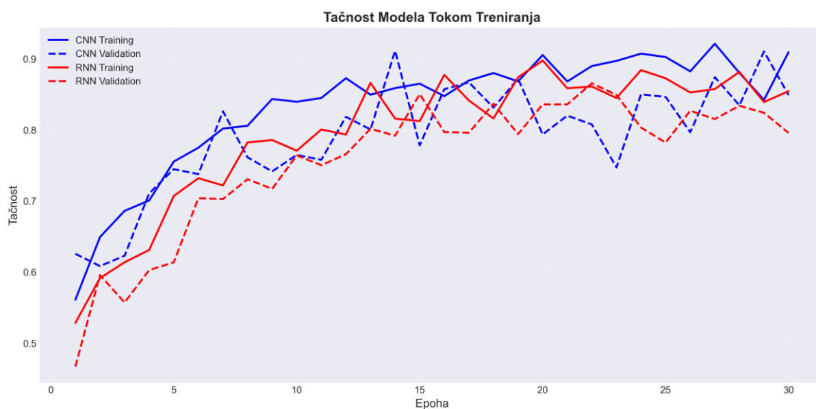
Slika 4: Uporedni prikaz tačnosti CNN i RNN modela tokom treniranja. Plava linija predstavlja CNN model, crvena RNN model.
