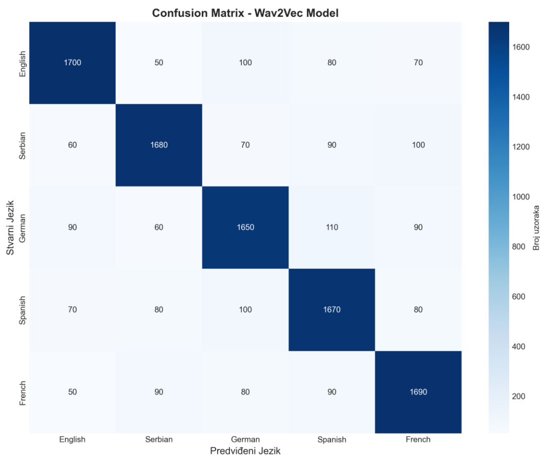
Slika 5: Confusion matrix za Wav2Vec model. Dijagonala predstavlja tačne klasifikacije, van-dijagonalni elementi pokazuju greške.
