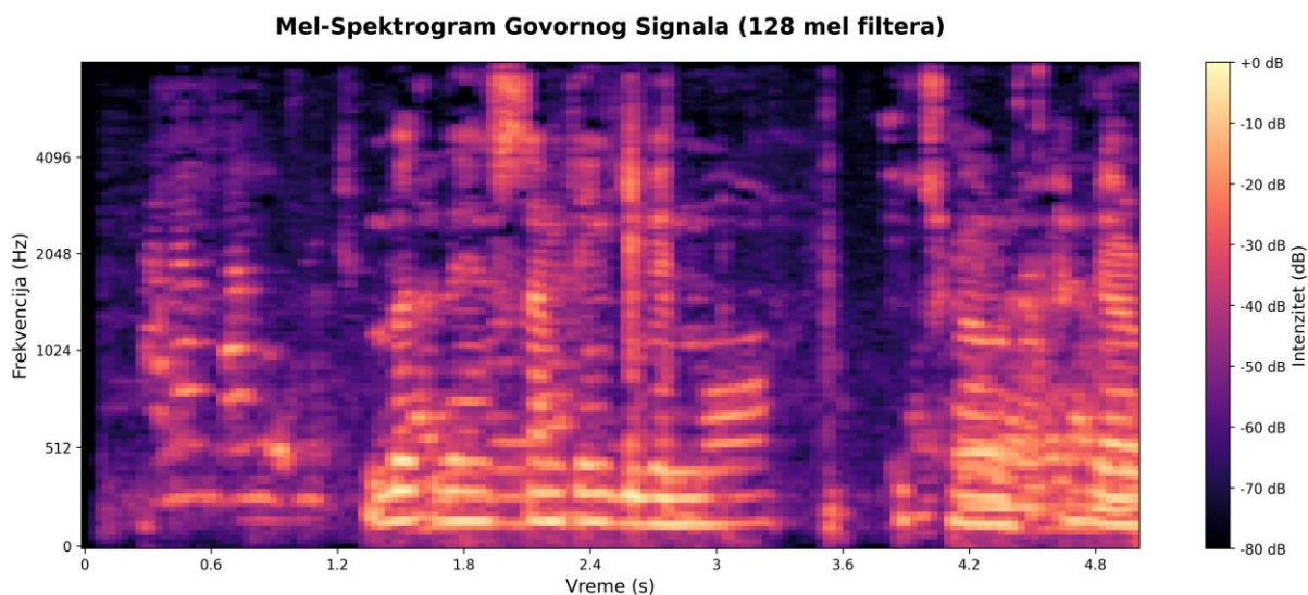
Slika 2: Mel-spektrogram govornog signala (128 mel filtera) prikazuje vremensko-frekventnu energetska distribuciju. Jasno vidljivi harmonici i formanti omogućavaju CNN modelima da automatski uče diskriminativne karakteristike različitih jezika.
